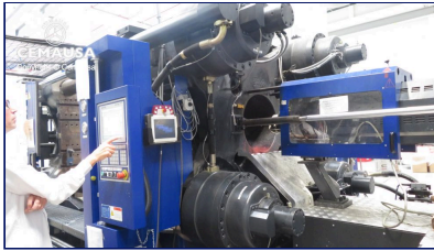
Inyectora termoplástico 1000 ton.
